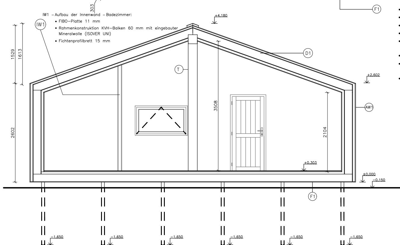
Schnitt B – B
